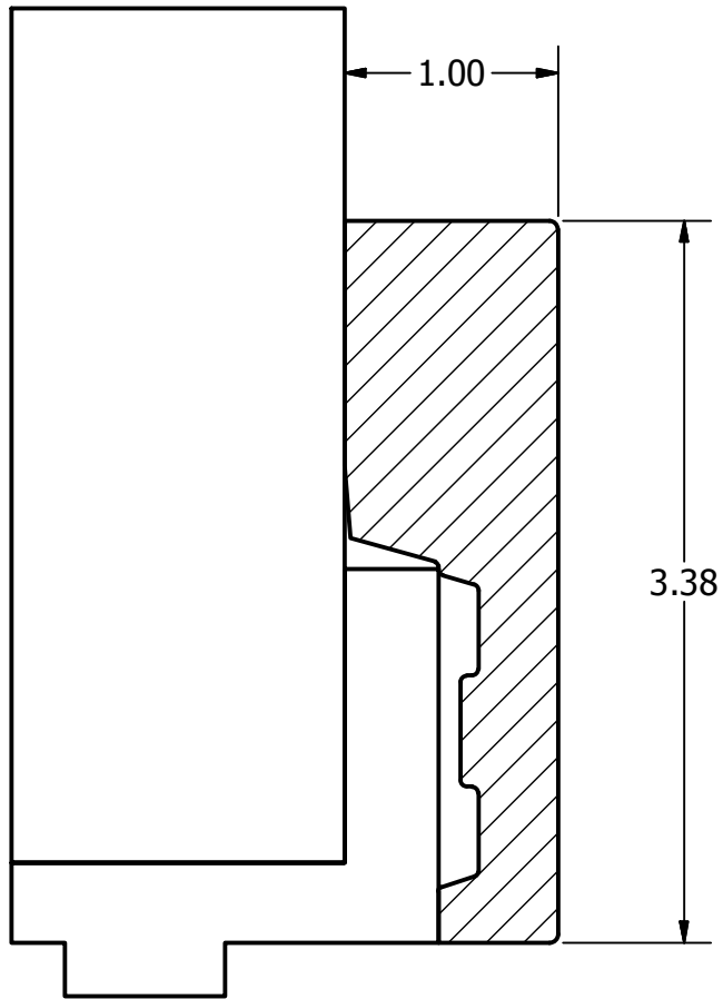
MG534P - PROFILE SCALE 1 : 1
